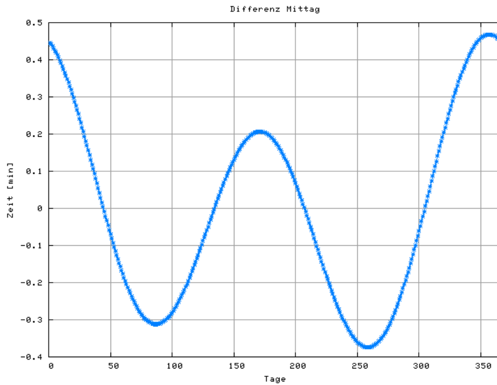
Bild 3: Differenz der Mittagszeiten
