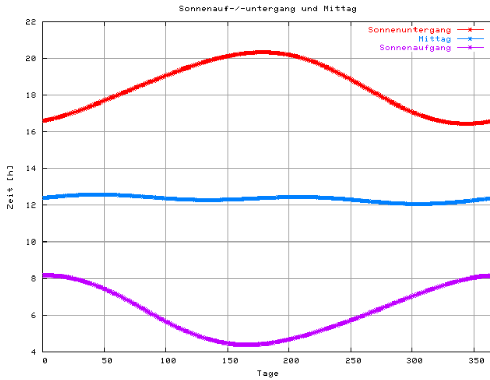
Bild 1: Sonnenauf-/untergang und Mittag
