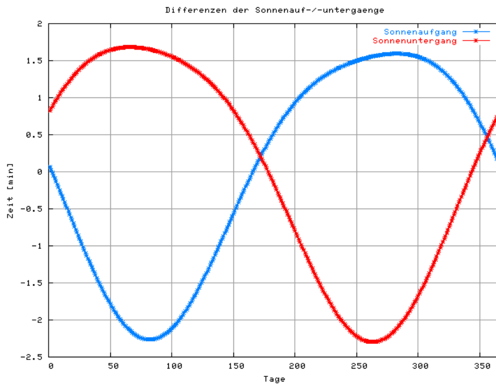
Bild 4: Differenz der Sonnenauf- und -untergänge
